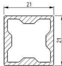
Vertikalni profil Vertical profile
