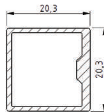
Horizontalni profil Horizontal profile
