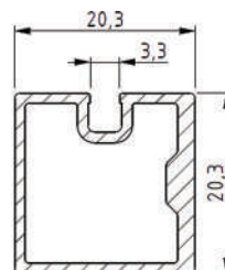
Profil za drsna vrata Sliding door profile
