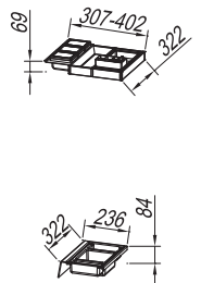
● ZG 350, SP 350 Drawer organizer Schublade Veranstalter Организатор ящик Fiókrendező
