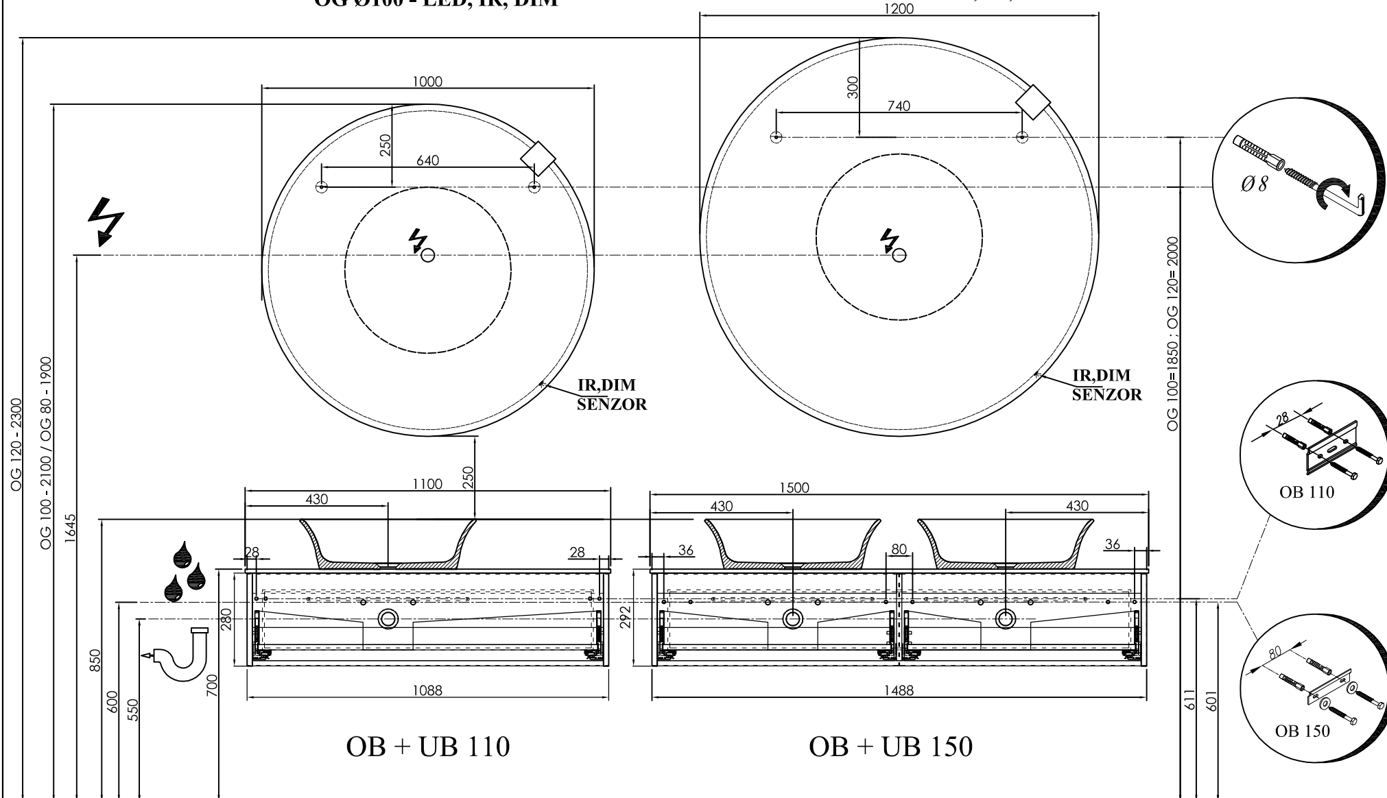
OG Ø120 - LED, IR, DIM
